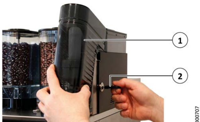
Rys. 53: Usuwanie osłony systemu instant
