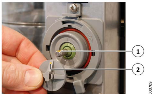
Rys. 56: Nakładanie koła miksera
