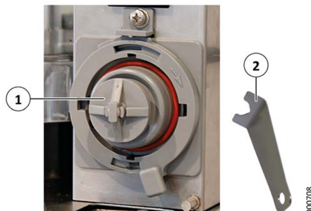
Rys. 55: Zdejmowanie koła miksera
