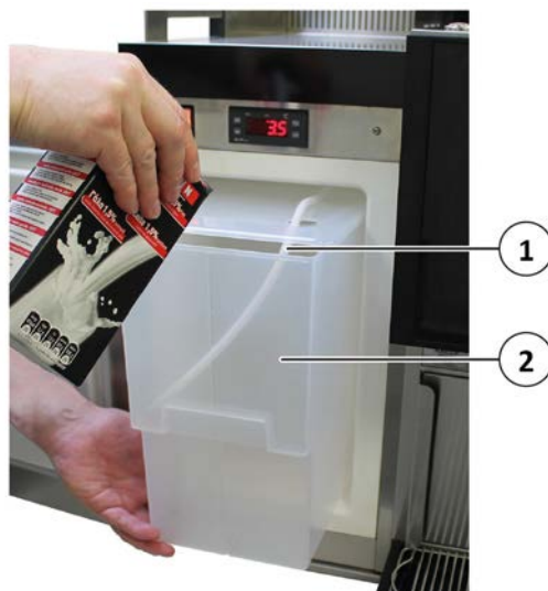
Rys. 10: Napełnianie pojemnika na mleko
