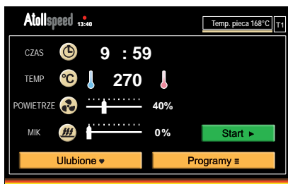
Ekran startowy
