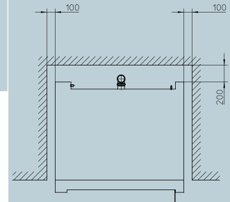
Rzut górny
