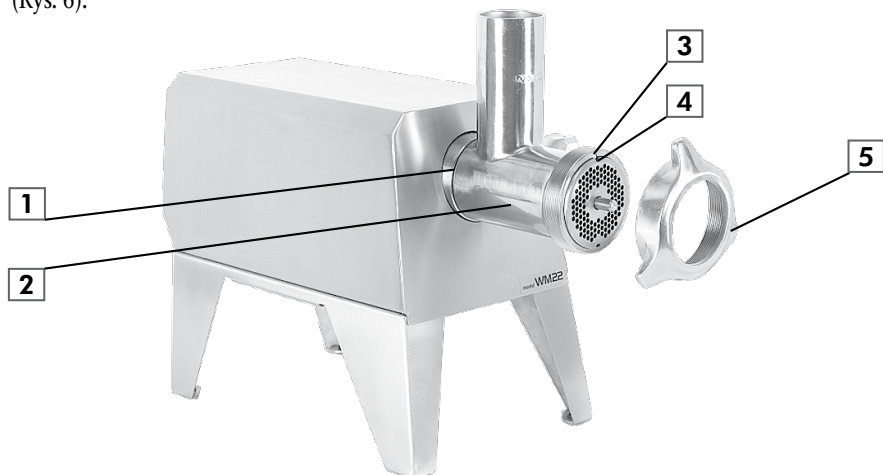
Rys. 6. Prawidłowe zamontowanie obudowy ślimaka w jednostce napędowej.
